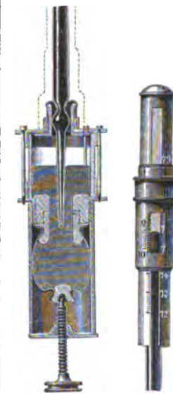
Č. 453. Barometr Fortinův.
